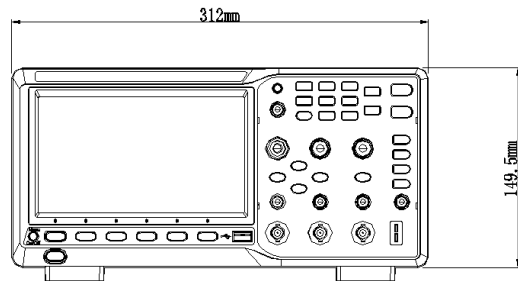
图 1 正视图
