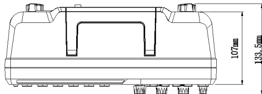
图 2 俯视图
